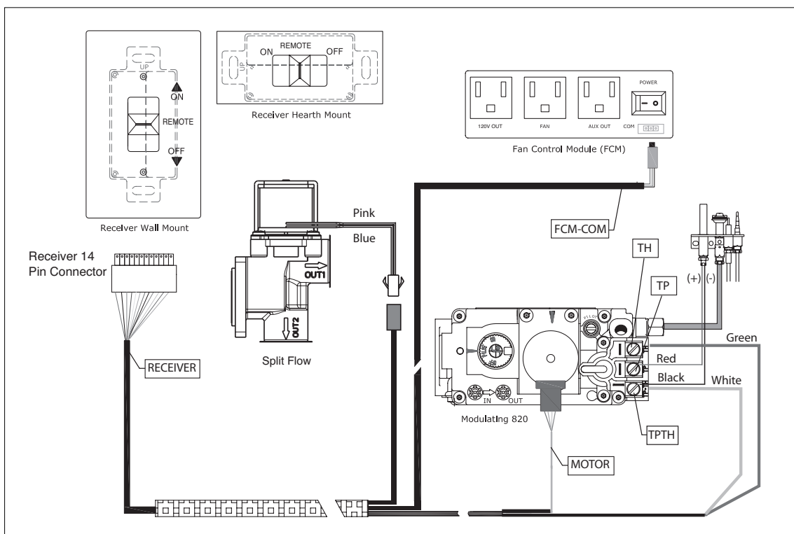
Fig. 2: Wiring diagram.
